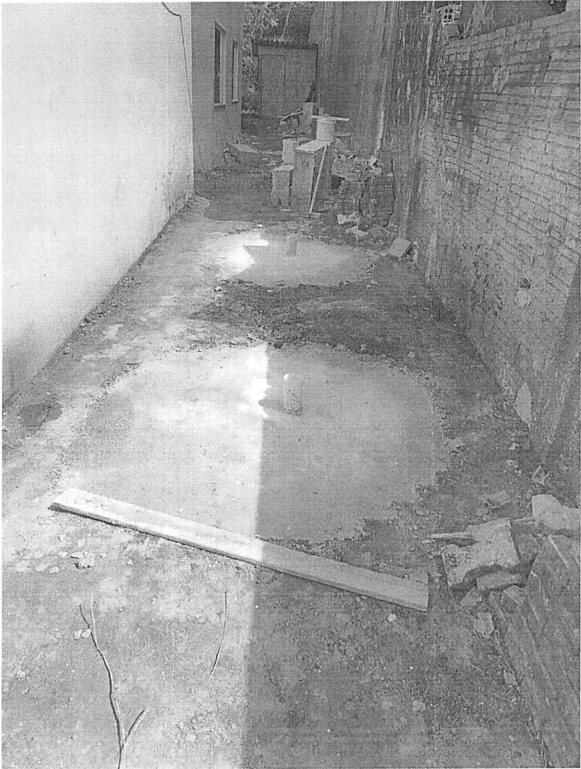
Imagem 2 – fossa e sumidouro.
